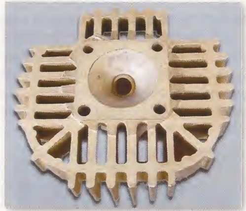
Vista inferior de la culata
